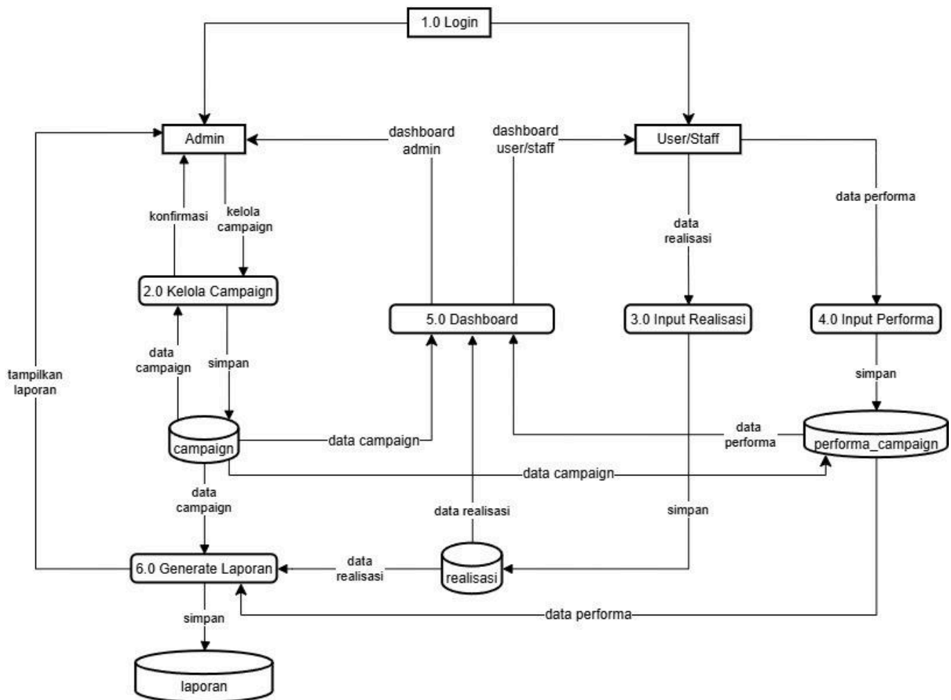
Proses DFD Ivl1
